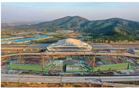
这是沪宁沿江高铁江阴站站房(4月10日摄)。近日,江阴站站房装饰装修作业已进入收尾阶段。 新华社记者季春鹏摄
