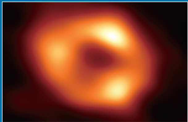
▼这是2022年5月12日包括中国在内的全球多地天文学家同步公布的银河系中心超大质量黑洞首张照片。 新华社发(事件视界望远镜供图)
