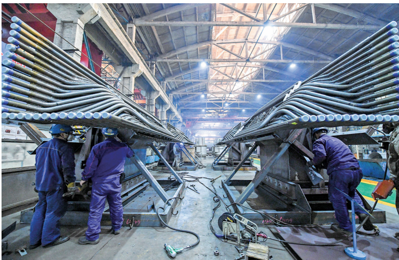
在哈电集团哈尔滨锅炉厂有限责任公司生产车间,工人在生产作业(二〇二三年十月二十四日摄)。新华社记者王松摄
