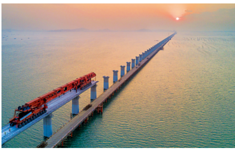
1月8日，在新建福厦铁路湄洲湾跨海大桥建设现场，“昆仑号”千吨级运架一体机在夕阳中作业。 新华社记者宋为伟摄
