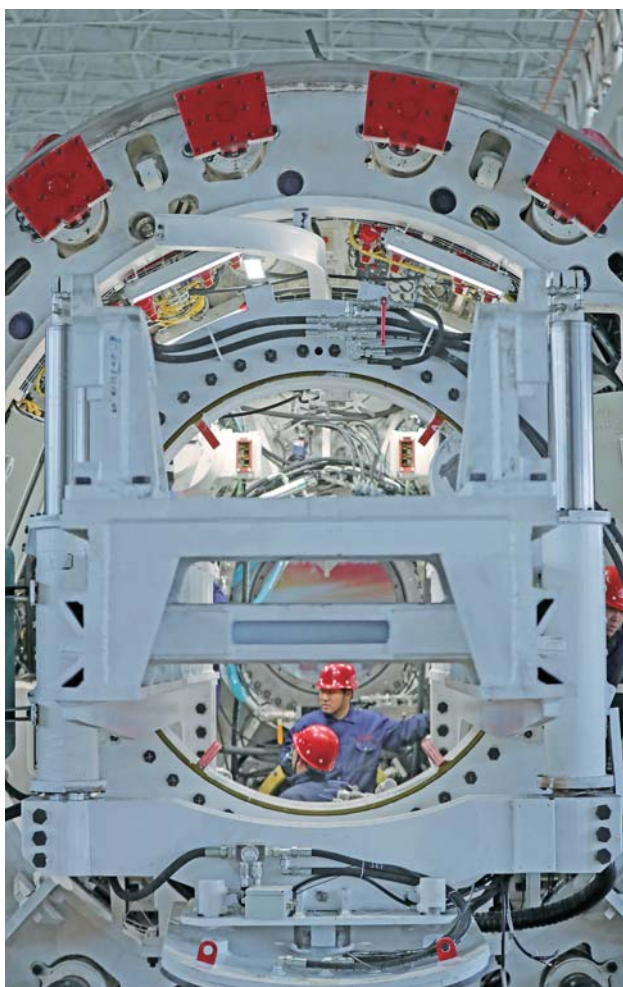
▲11月22日,辽宁三三工业有限公司工程技术人员在车间生产盾构机。新华社记者杨青摄
